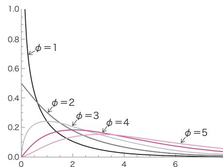
図表 3.7 自由度 \phi の \chi^2 分布
